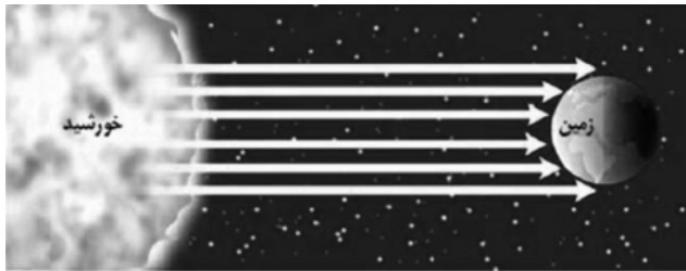
شکل ۲. تصویر نادرست اندازه و فاصله زمین تا خورشید بدون در نظر گرفتن مقیاس
